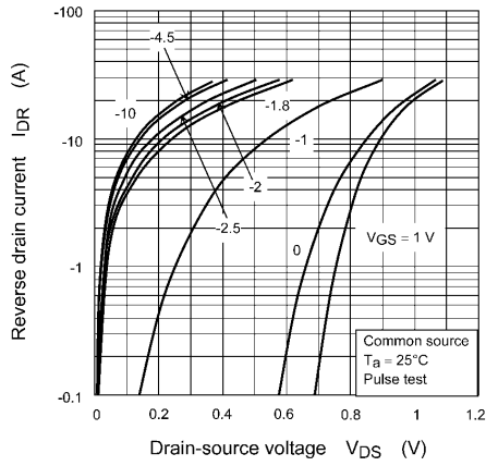
Fig. 8.7 I_{DR} - V_{DS}
