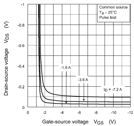
Fig. 8.4 V_{DS} - V_{GS}
