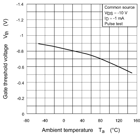
Fig. 8.9 V_{th} - T_a
