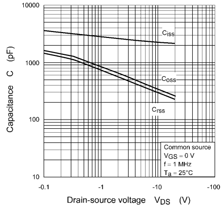
Fig. 8.8 Capacitance - V_{DS}
