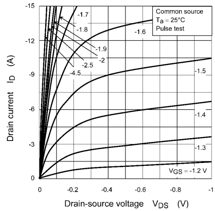
Fig. 8.2 I_D - V_{DS}
