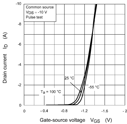
Fig. 8.3 I_D - V_{GS}
