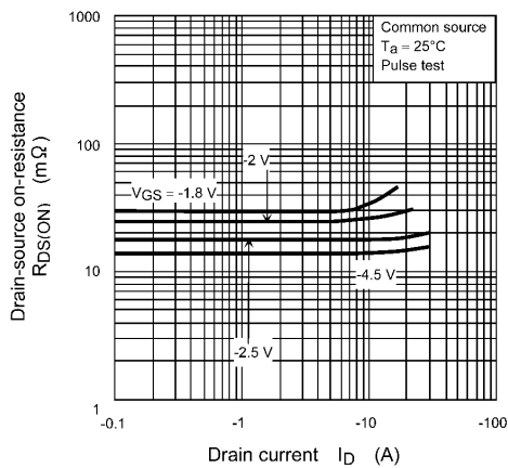
Fig. 8.5 R_{DS(ON)} - I_D
