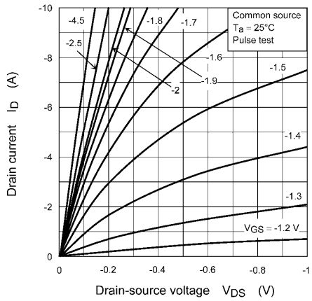
Fig. 8.1 I_D - V_{DS}
