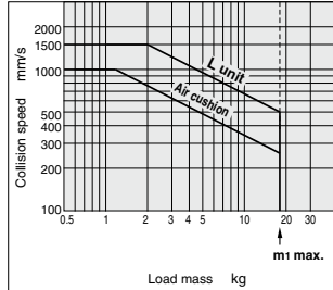
MY1C16
