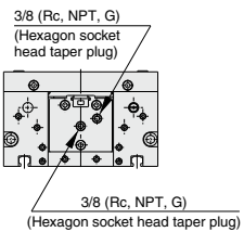
MY1HT□G
