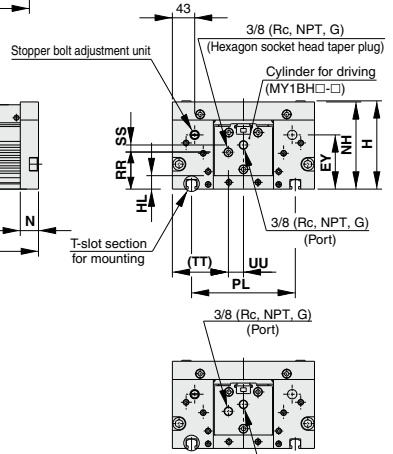
MY1HT□G
