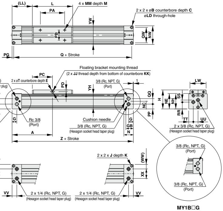
MY1B□G
