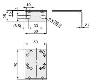
L-bracket
