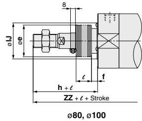
ø80, ø100
