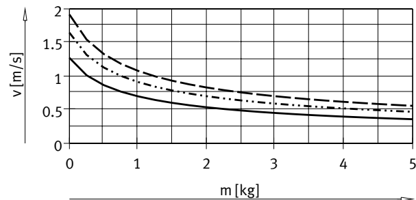
Piston ø 16
