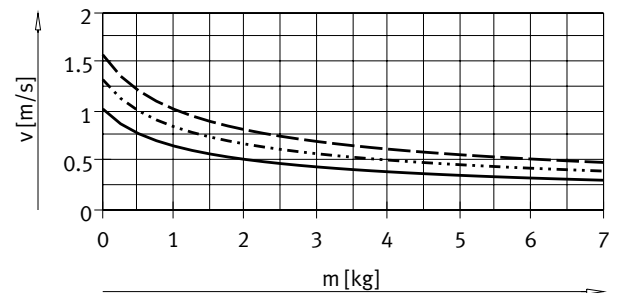
Piston ø 20
