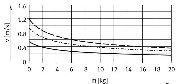
Piston ø 32
