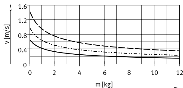
Piston ø 25
