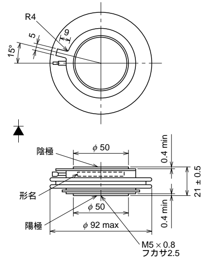
外形図
