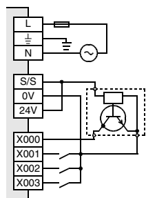
Датчик, переключающий на минус (Sink)
