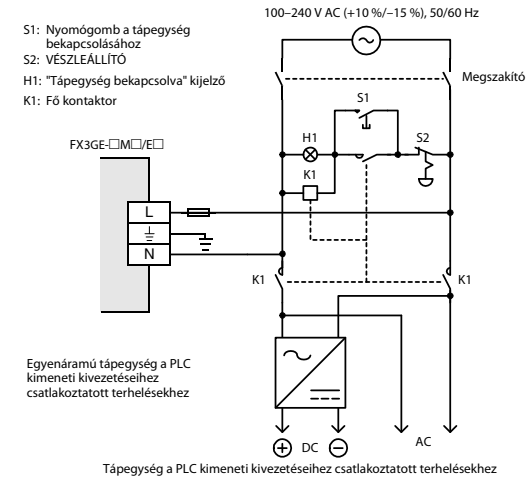
Tápegység a PLC kimeneti kivezetéseivel csatlakoztatott terhelésekhez
