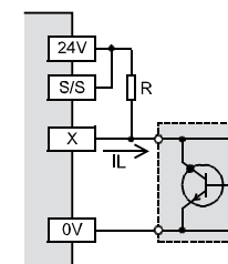
переключение на минус (Sink)
