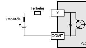
Tranzisztor kimenet (nyelő)
