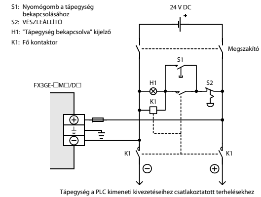
Tápegység a PLC kimeneti kivezetéseivel csatlakoztatott terhelésekhez
