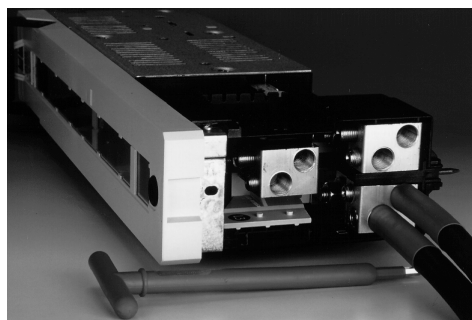
Bild 7 Baugröße 1, Sicht auf 3 Doppelklemmen, 2 Kabel angeschlossen
