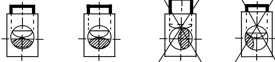
Bild 4: Positionierung eines sektorförmigen Kabels in der Klemme
