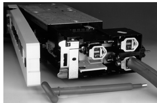
Bild 6: Baugröße 1, Sicht auf 3 Einfachklemmen, 1 Kabel angeschlossen
