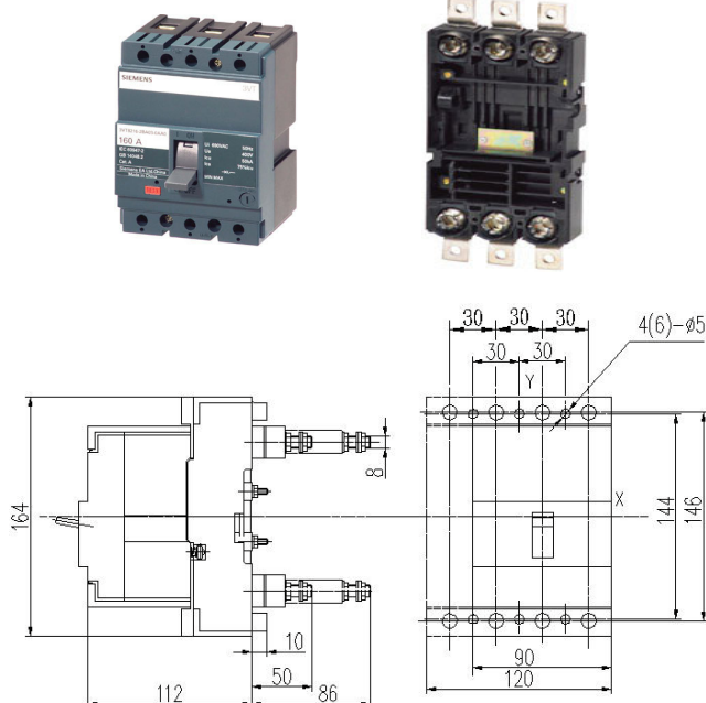
(5) Versão de encaixe do disjuntor de potência VT160
