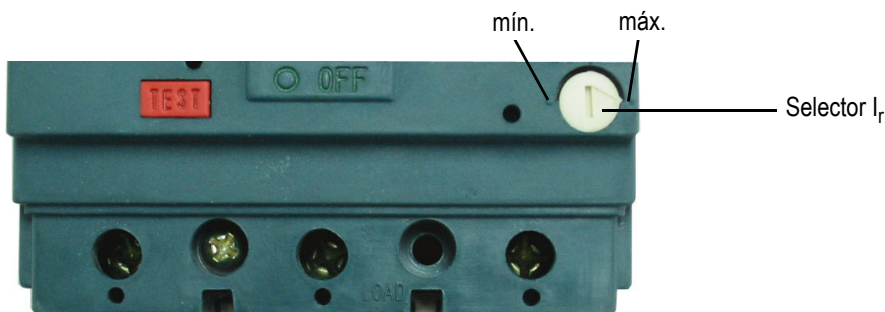
(19) Unidad de disparo termomagnético del VT160 con I_r ajustable
