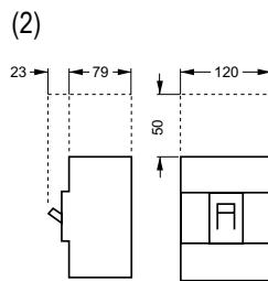
灭弧室上方所需空间 与紧贴接地元件以及非绝缘导电部件的最少空间
