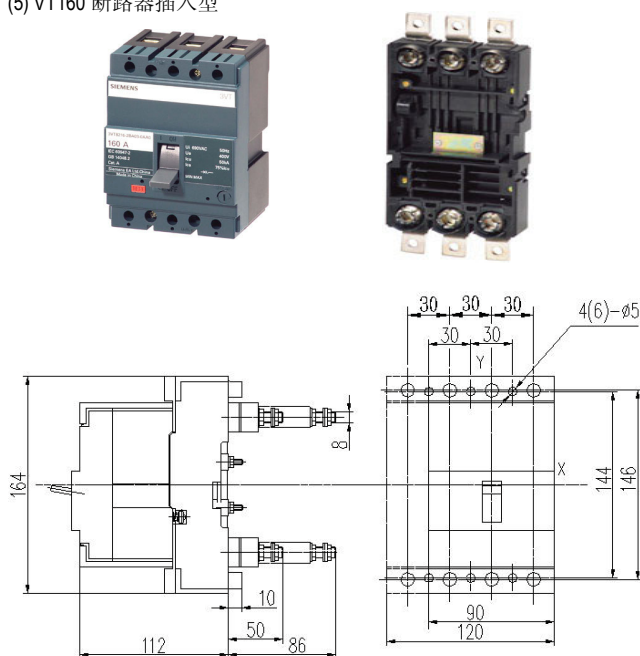
(5) VT160 断路器插入型
