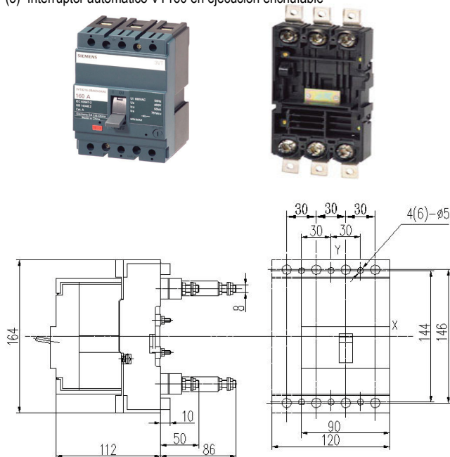
(5) Interruptor automático VT160 en ejecución enchufable
