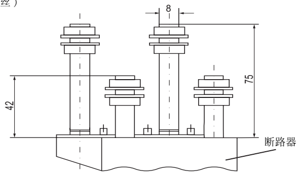
后夹板 (螺丝)
