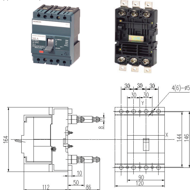
(5) Versione a spina dell'interruttore automatico VT160
