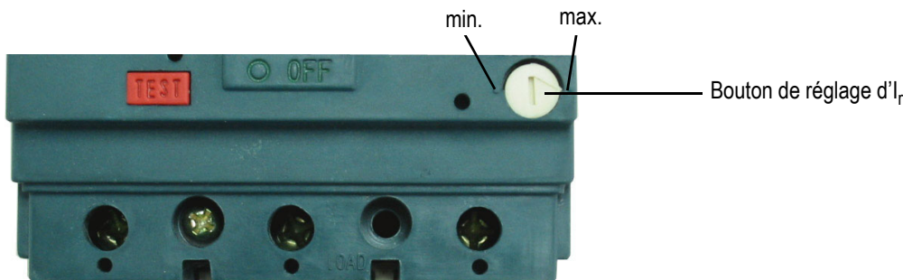
(19) Unité de déclenchement thermomagnétique du VT160, I_r réglable
