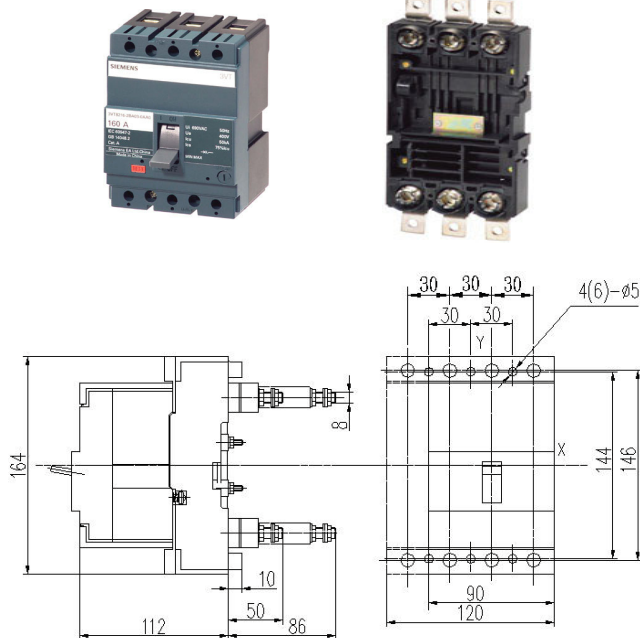
(5) штекерный вариант силового выключателя VT160
