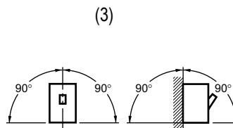
灭弧室上方所需空间 与紧贴接地元件以及非绝缘导电部件的最少空间
