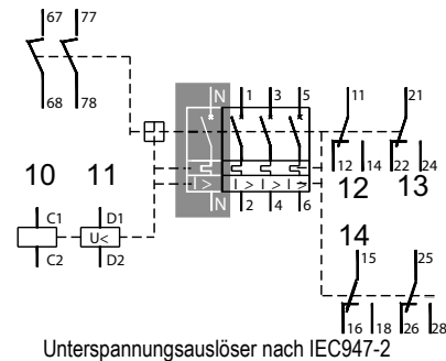
Unterspannungsauslöser nach IEC947-2
