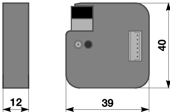
Fig. 7 : Dimensions BI-F-4.0.1
