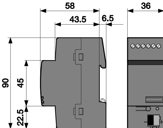
Fig. 8 : Dimensions BI-M-4.0.1
