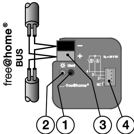
Fig. 3 : Vue d'ensemble de l'entrée binaire double à encastrer
