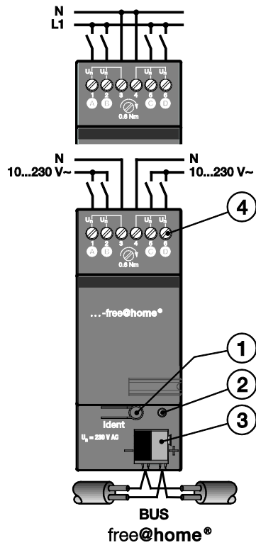
Fig. 5 : Vue d'ensemble de l'entrée binaire quadruple MDR
