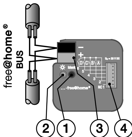
Fig. 4 : Vue d'ensemble de l'entrée binaire quadruple à encastrer
