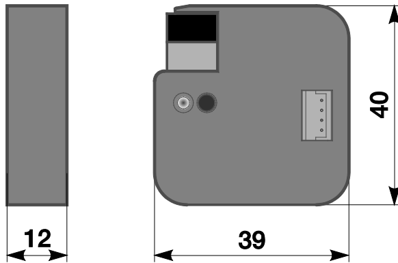
Fig. 6 : Dimensions BI-F-2.0.1
