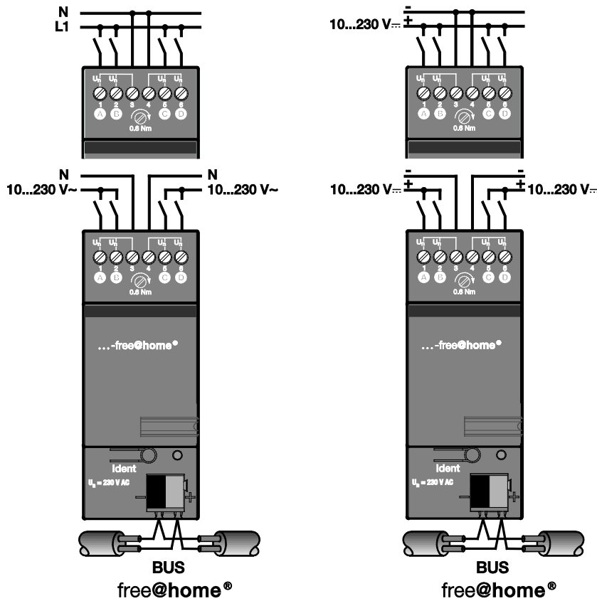
Fig. 11 : Raccordement électrique BI-M-4.0.1
