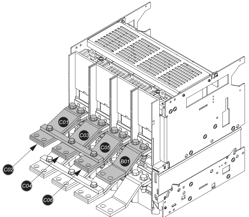
TERMINALE SUPERIORE UPPER TERMINAL OBERE ANSCHLUSS BORNE SUPÉRIEURE TERMINALES SUPERIOR
