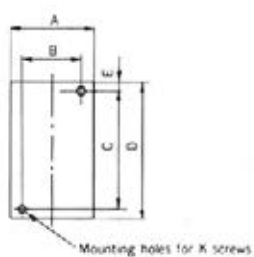
H80C-L-H150C-L
