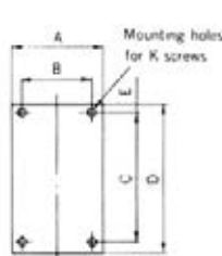
H200C-L-H600C-L
