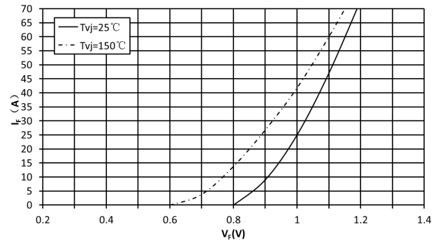
正向偏压特性 二极管,整流器 (典型) forward characteristic of Diode, Rectifier (typical) I_F = f(V_F)
