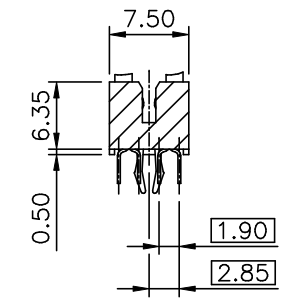
SEC: A-A SCALE 2:1
