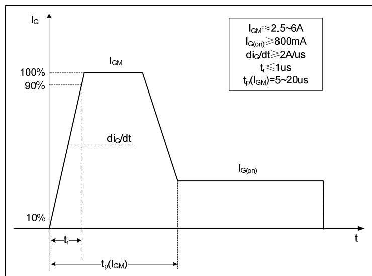
图9. 门极触发推荐波形
